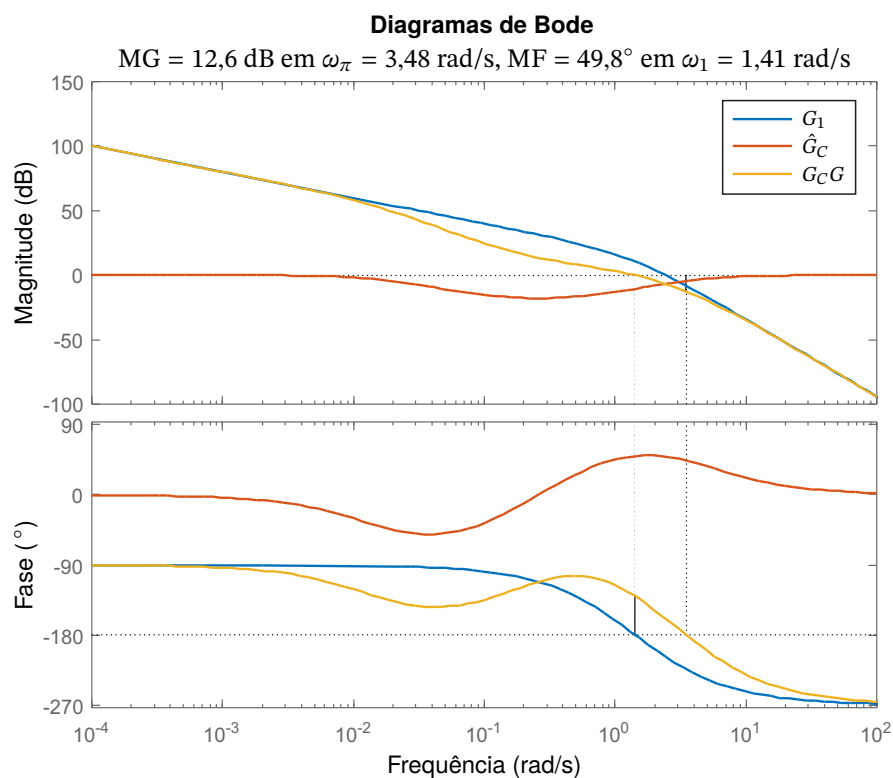
Figura 3.1 – Resposta em frequência de malha aberta
